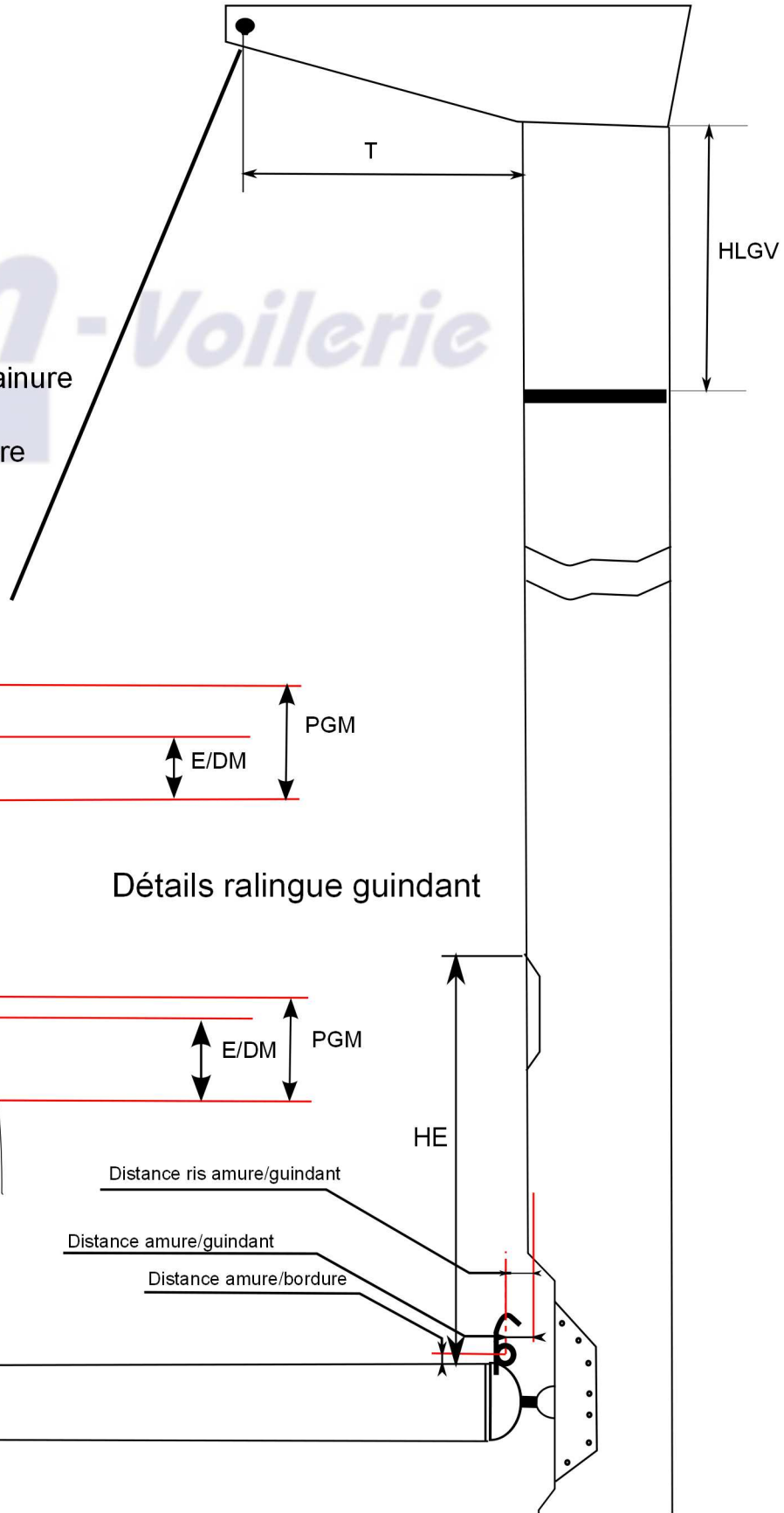
Détails amure
